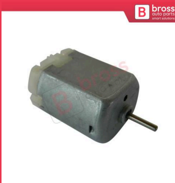
BGE16 Side Mirror Folding Motor for Mabuchi FC-280PC-22125 12 Volt BMW Mini Rover Chrysler Freelander Evoque Liberty
